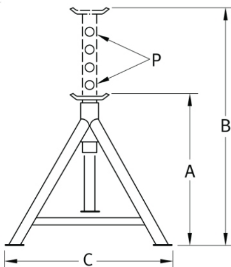
Desenho dimensional
