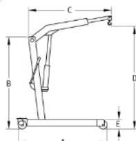
Desenho dimensional
