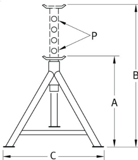
Desenho dimensional
