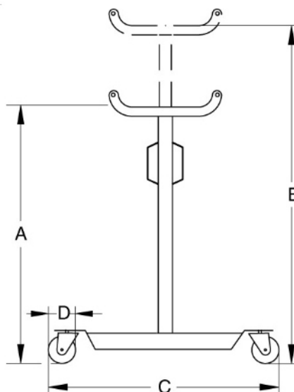
Desenho dimensional
