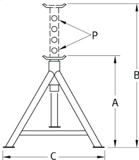
Desenho dimensional
