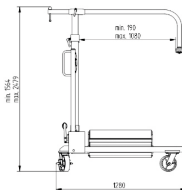
Desenho dimensional
