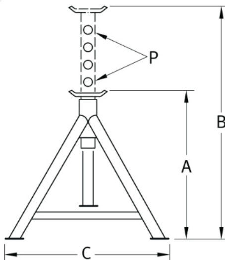
Desenho dimensional
