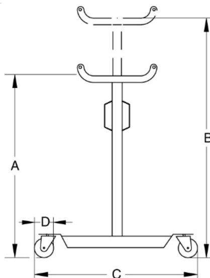
Desenho dimensional
